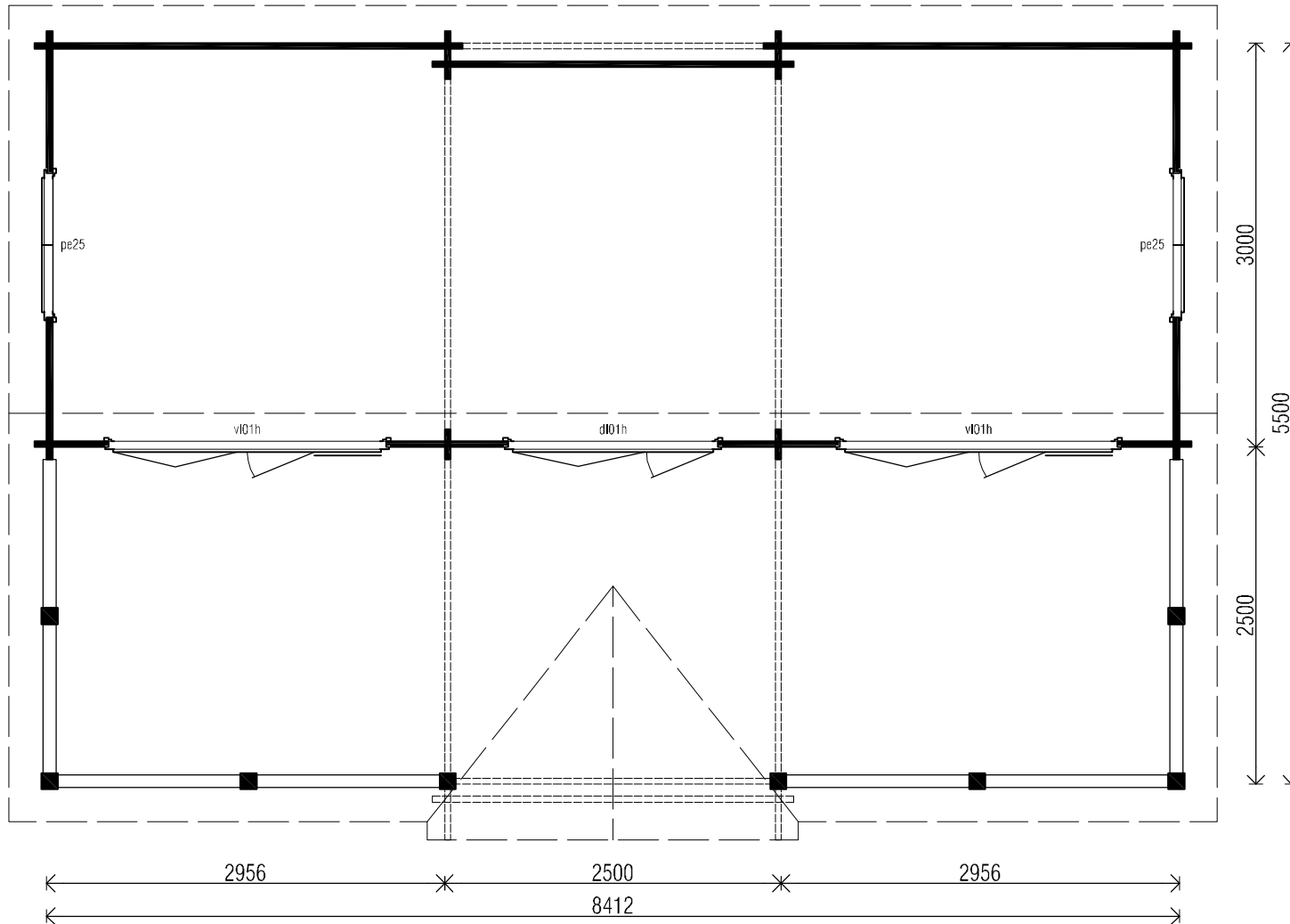
plattegrond / plan
