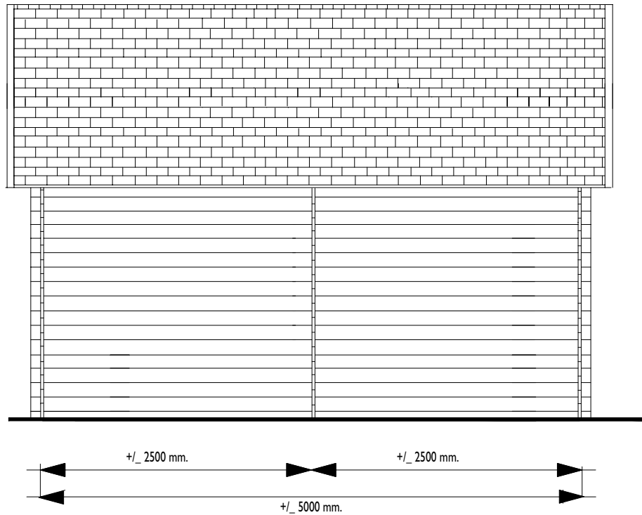
Zij aanzicht Seiten Ansicht Side view
