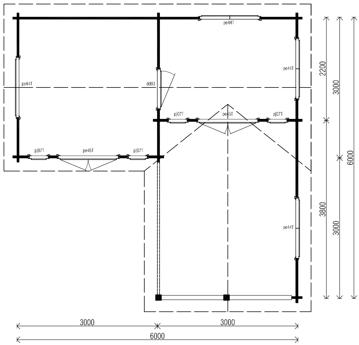
plattegrond / plan
