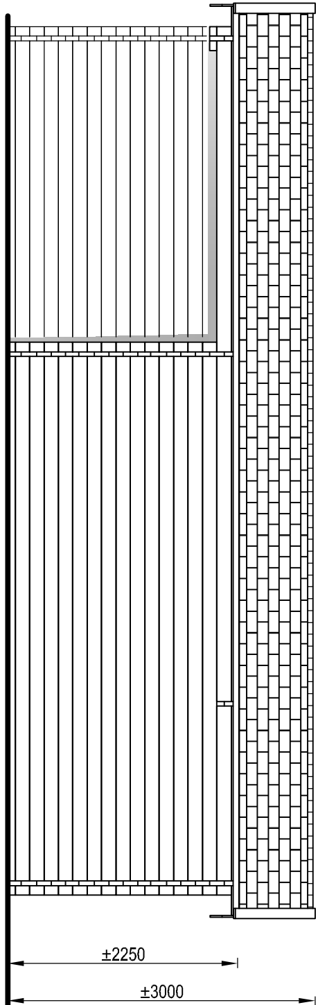
Zij aanzicht - Seiten Ansicht - Side view
