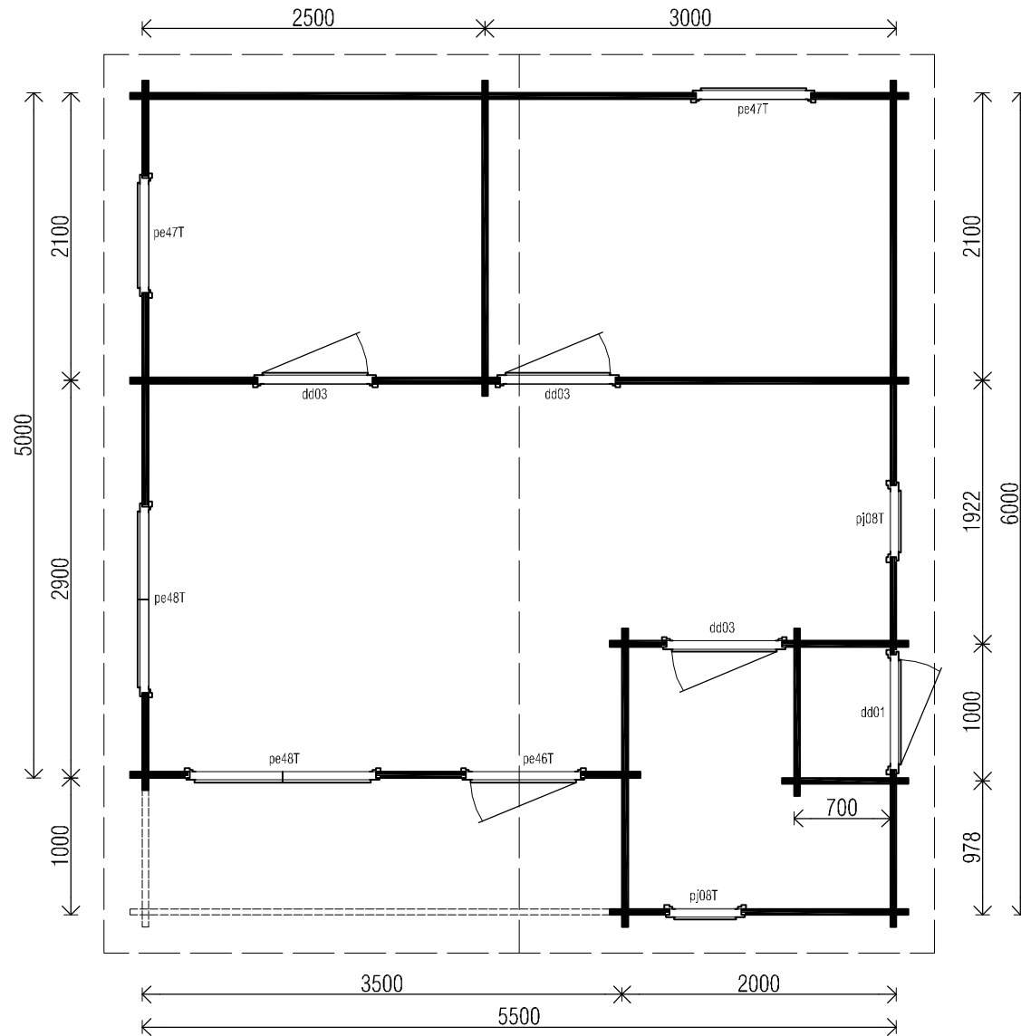
plattegrond / plan
