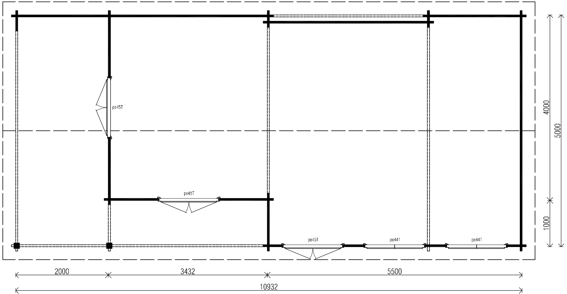
plattegrond / plan
