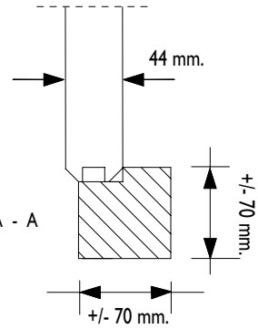
Zij aanzicht Seiten Ansicht Side view
