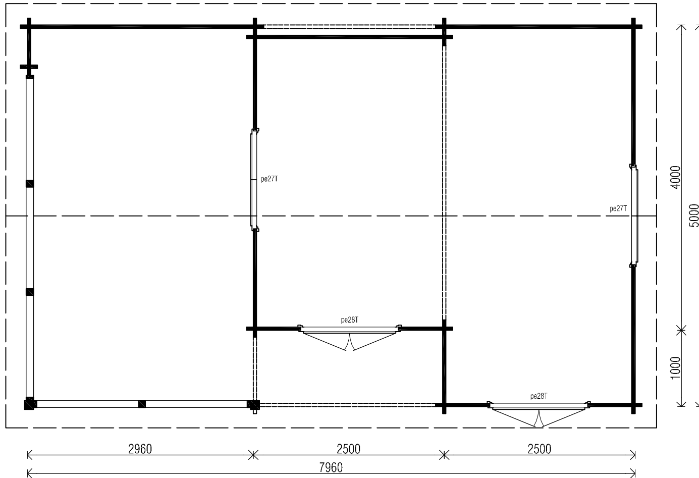
plattegrond / plan
